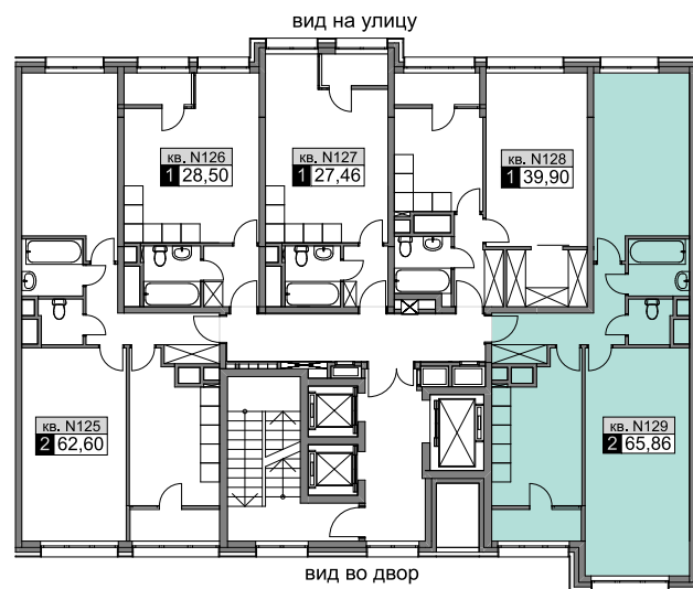
ПЛАН СЕКЦИИ | ЭТАЖ 4, СЕКЦИЯ 3
